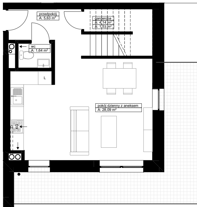
rzut piętra +3
