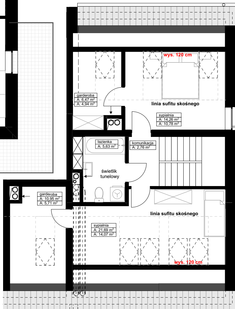
rzut poddasza +4
